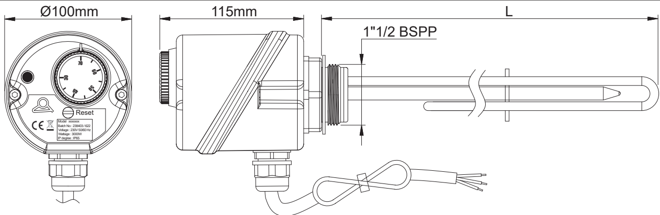
1-poliger 230V-Heizer
